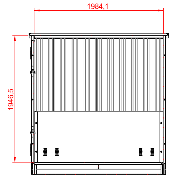
SECTION A-A SCALE 1 : 35
