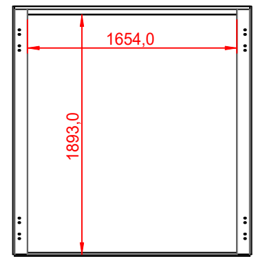
DOUBLE DOOR DIMENSIONS 1893 x 1654 x 35
