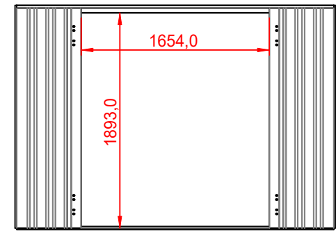
DOOR DIMENSIONS 1893 x 1654 x 35
